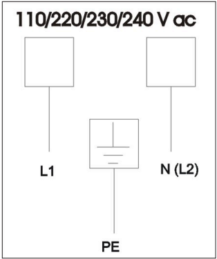
Schema elettrico
